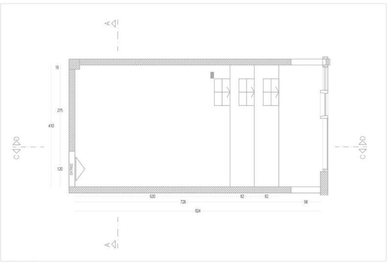
PLAN SALLE 05
