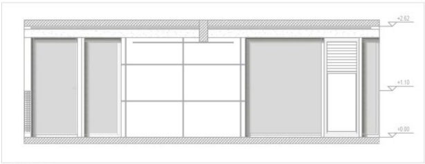
ELEVATION A-A
