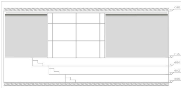
ELEVATION B-B
