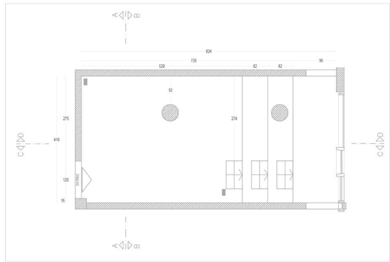
PLAN SALLE 05
