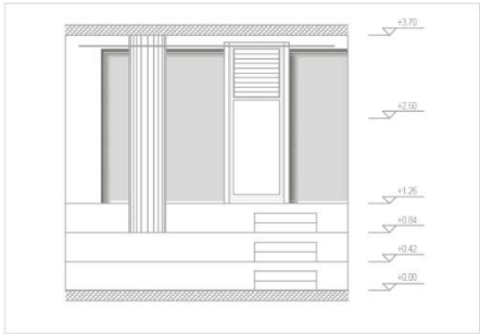
ELEVATION B-B
