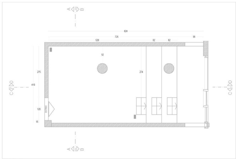
PLAN SALLE 05
