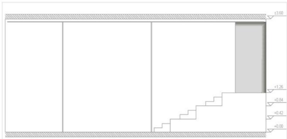
ELEVATION A-A
