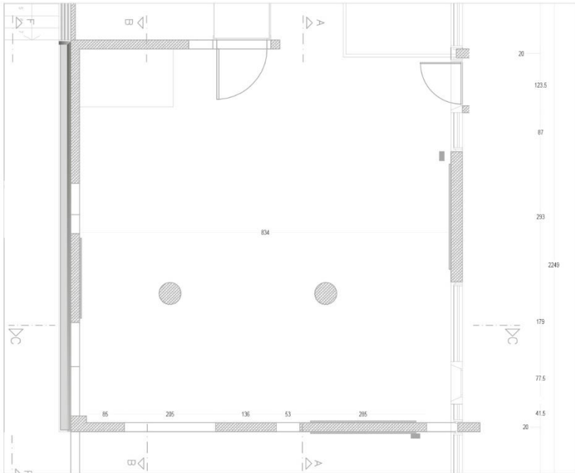
PLAN SALLE 07
